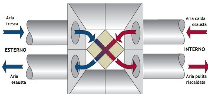
Ricambio d'aria con recupero di calore
